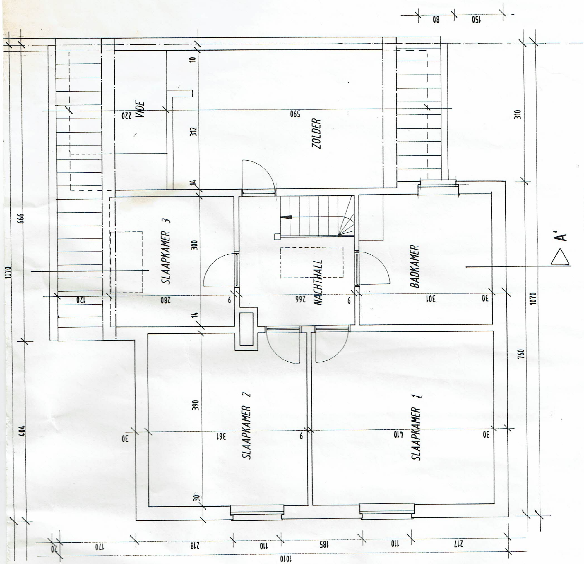
VERDIEPINGSPLAN
