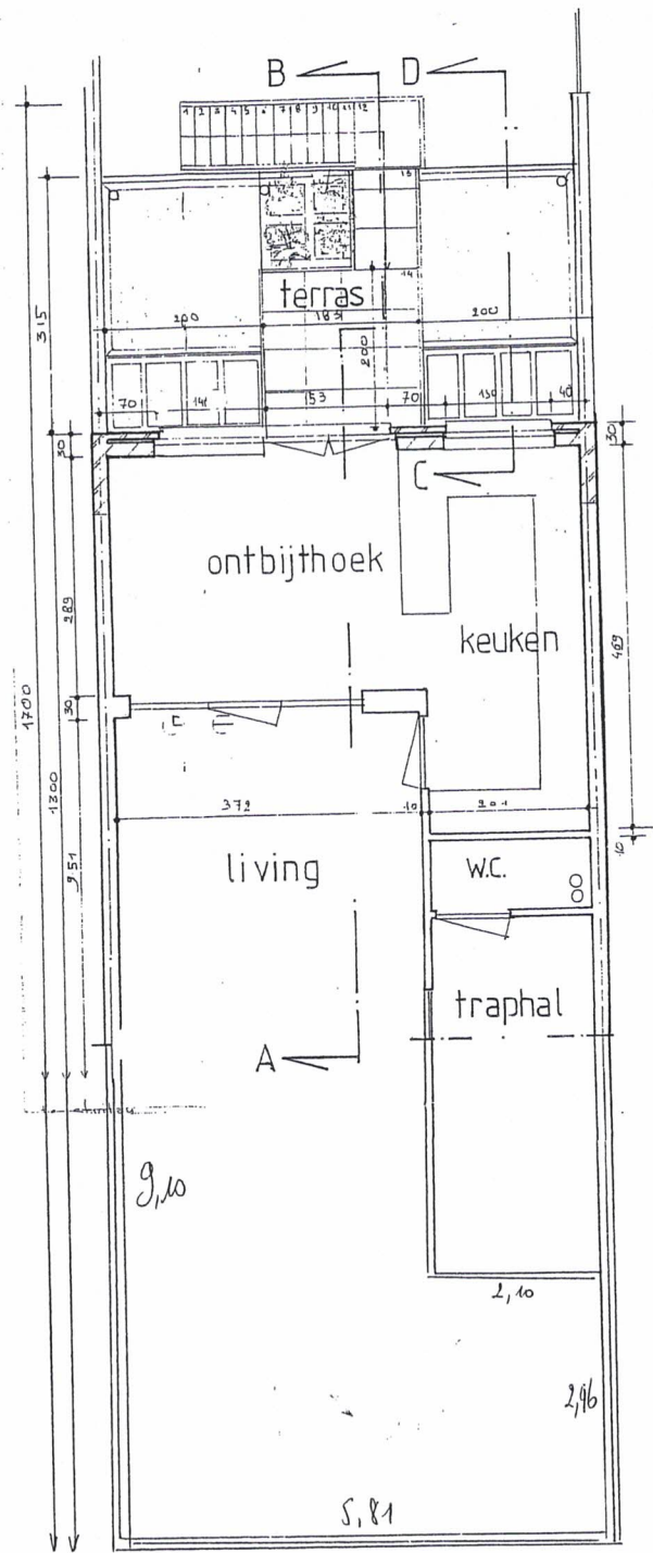
1 e VERDIEPING
